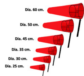
อุปกรณ์ทิศทางลม
